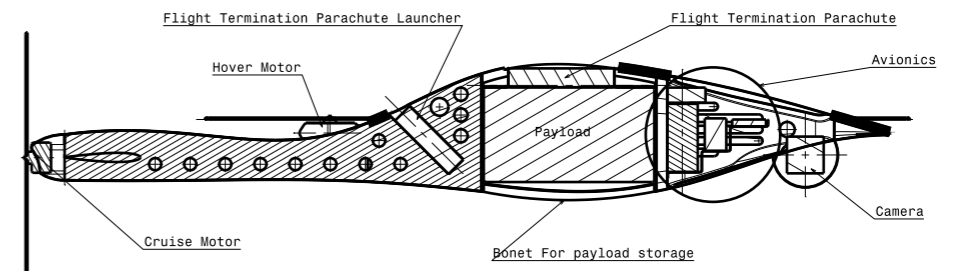
Section view A-A Scale: 1:7
