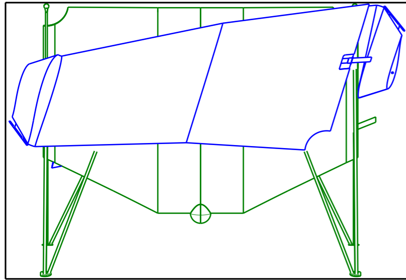
Bottom view Scale: 1:20
