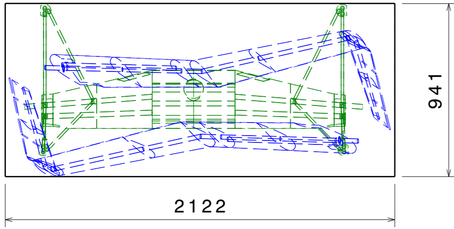
Front view Scale: 1:20
