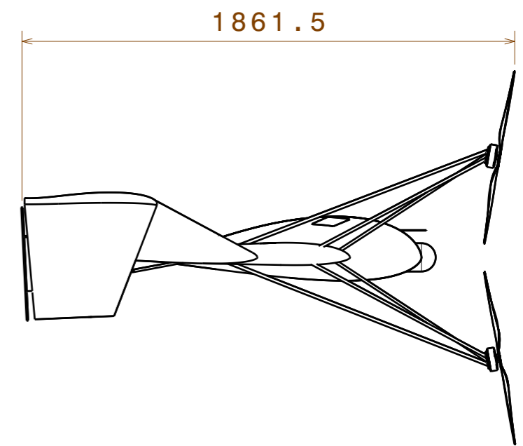
Left view Scale: 1:20
