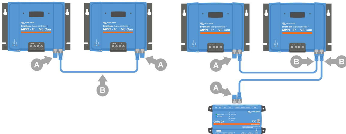
A: VE.Can terminator - B: RJ45 UTP cable.
