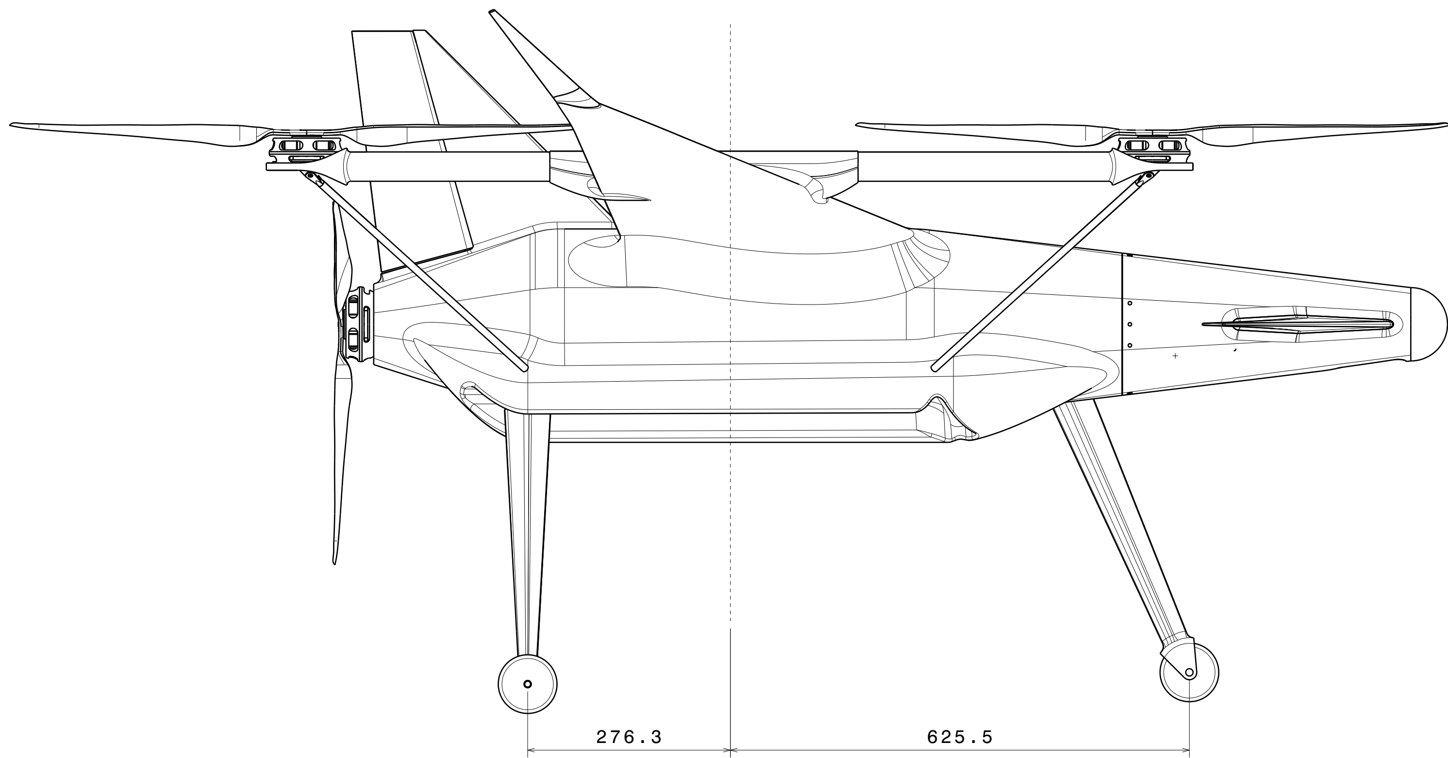
LATERAL VIEW Scale: 1:5
